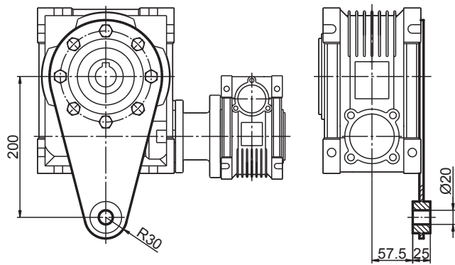
Ramię reakcyjne
