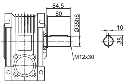
Wał zdawczy jednostronny
