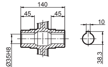
Tuleja zdawcza
