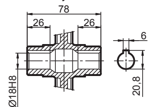
Tuleja zdawcza
